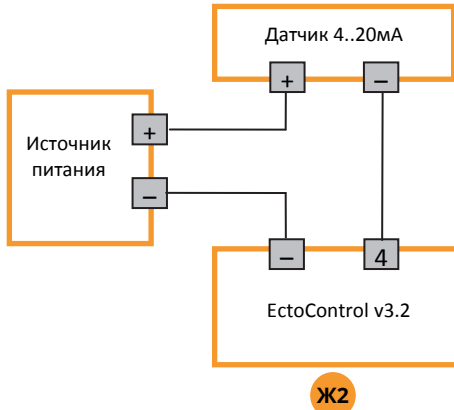
Питание датчика от стороннего источника питания
